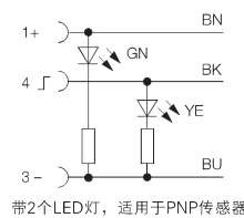
带2个LED灯，适用于PNP传感器
